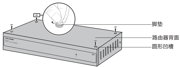
图2-1 桌面安装示意图
