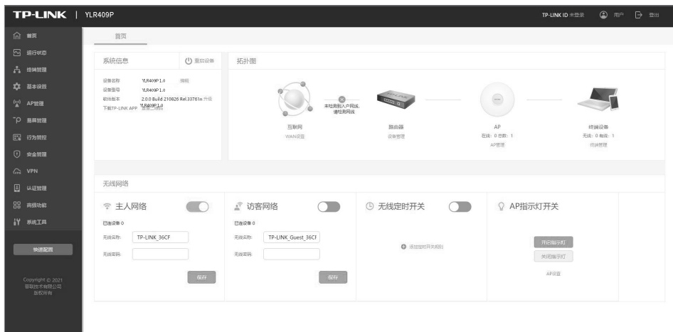
图4-11 首页
